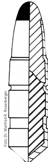
Geschossaufbau: Das Brenneke TUGnature.
